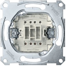
Anahtar mekanizması
